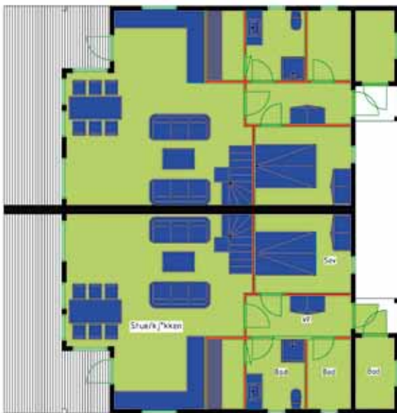
PLAN HOVEDETASJE Bebygd areal pr. enhet. 76,6 kvm (totalt 153,2 kvm). Boareal pr. enhet. 124 kvm
